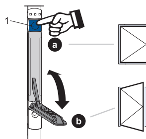
Bild 2: Stulpfenster
