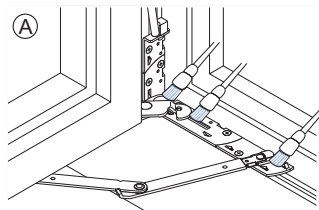
Bild 3: Ecklager
