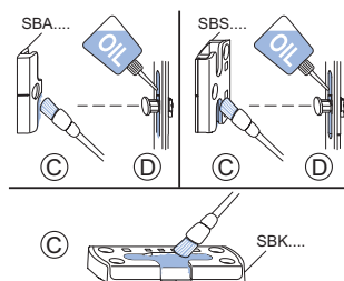
Bild 2: Schließbleche
